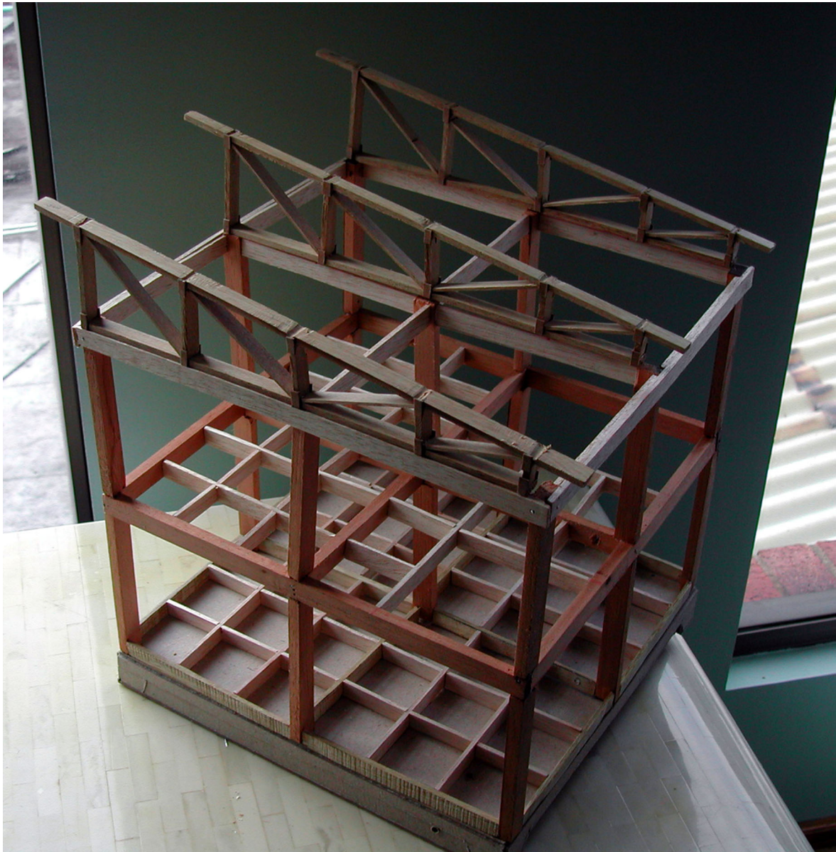
Estructura principal y secundaria, entramados
