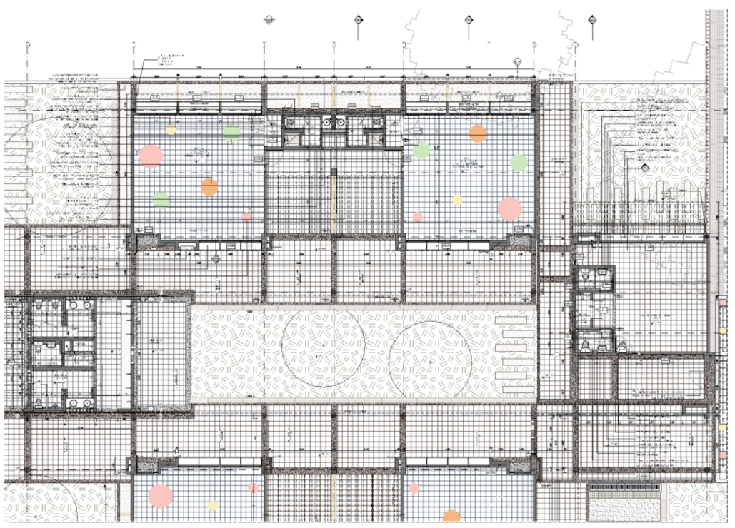
PLANTA BLOQUES PREESCOLAR
