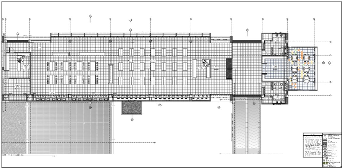
PLANTA EDIFICIO DE ACCESO
